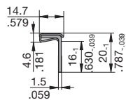
Plug-on cap, 1-pole Y 307 851 01
