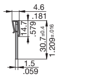
Plug-on cap, 1-pole Y 307 851 01
